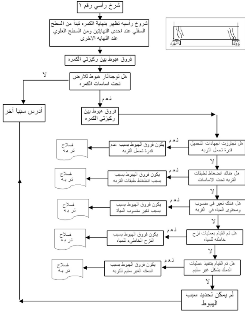
شكل (١) - شجرة القرارات لشروخ رأسي رقم ١-كمرات
